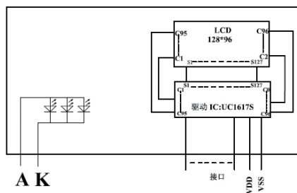
电路框图
