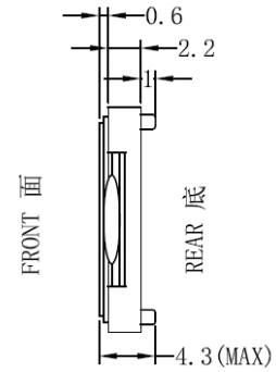
侧面图
