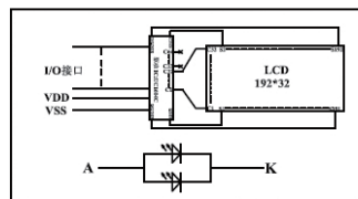
电路框图
