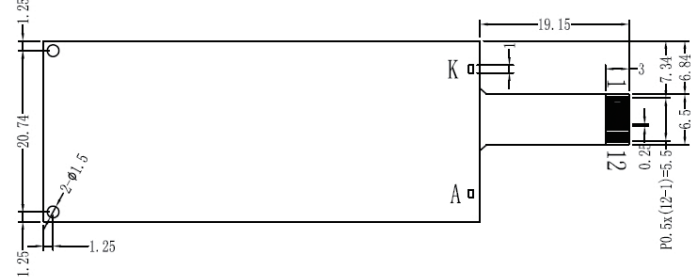
背面图
