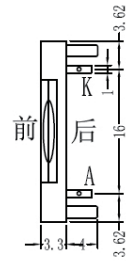
侧面图
