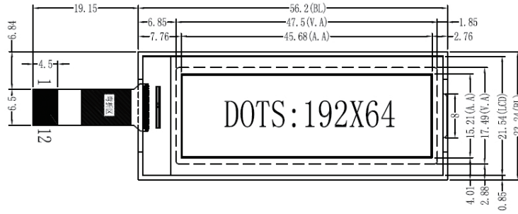
正面图
