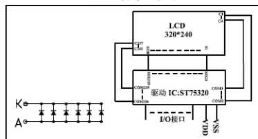
电路框图
