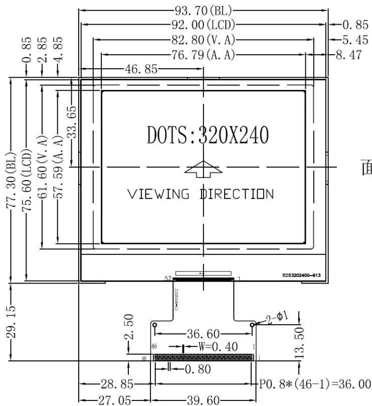
正面图
