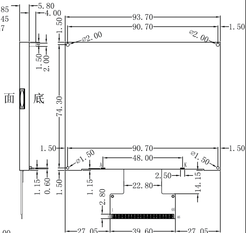
侧面图
